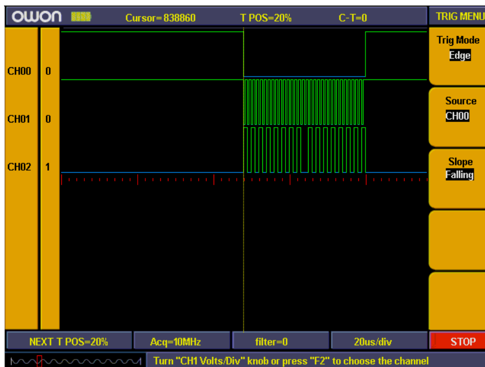
Fig.5-55: Edge trigger setting
